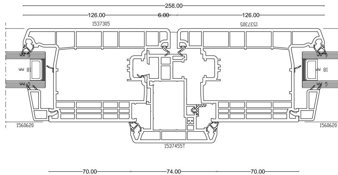
Sezione B - orizzontale
